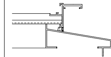
中棧フレーム(大) 端部断面
