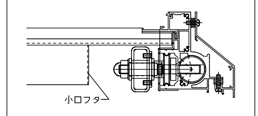
中棧フレーム(大) 端部断面
